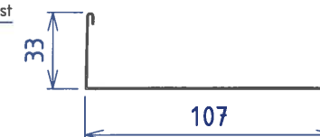
festeklips
