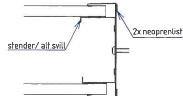
rammeprofil- slett
