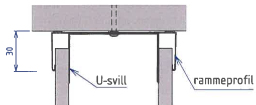
rammeprofil- vinkelst
