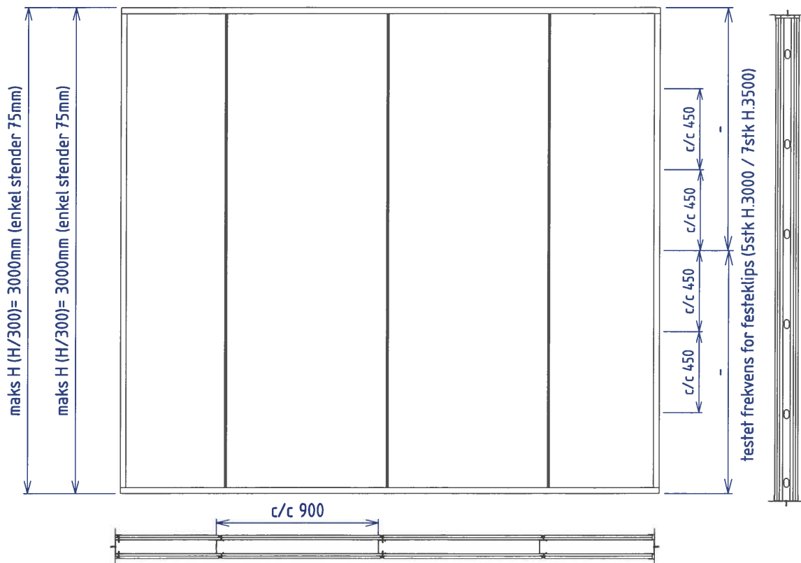
rammeprofil-slett
