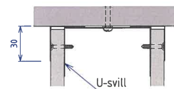
belistning- vinkelst
