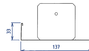
rammeprofil- m.flik
