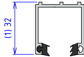
U-PROFIL (10-16,8 glass)
