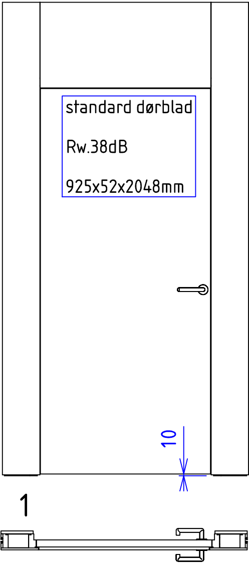
innadslående konstruksjon
