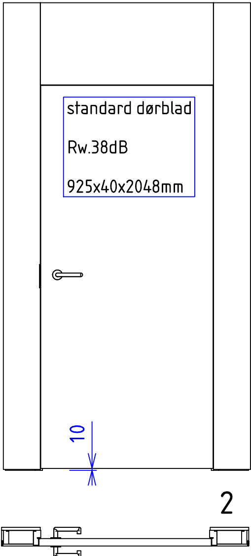
utadslående konstruksjon
