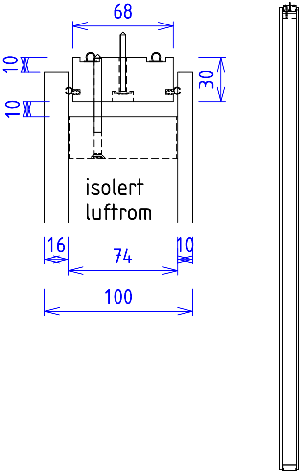
tilvalg: montasjeteleskop
