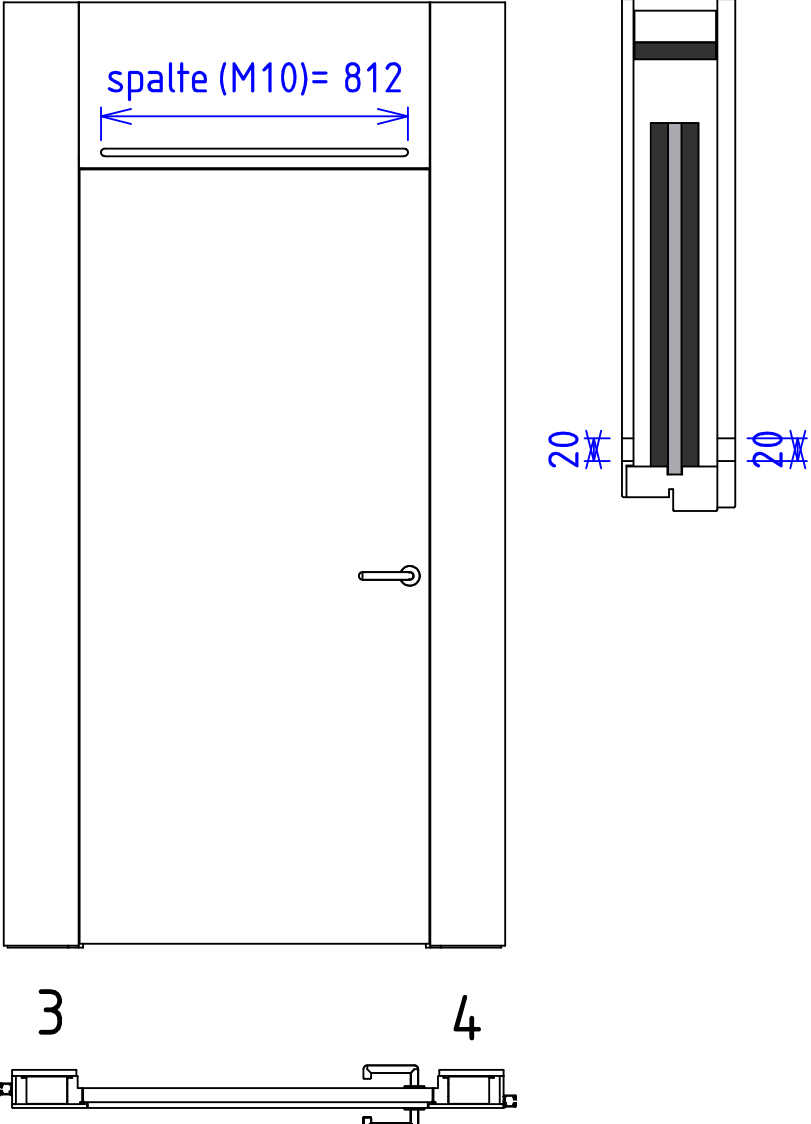
tilvalg: overluftgj.strømning
