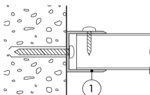
Montering til veggen i rommet.
